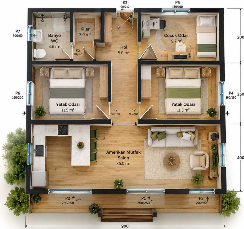
BULUT BEY EVİ - YALOVA ZEMİN KAT PLANI
